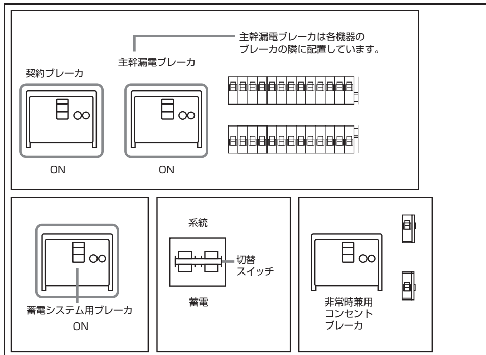
分電盤、ブレーカーの配置例 2
