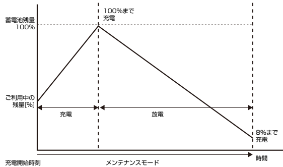
メンテナンスモード動作イメージ
