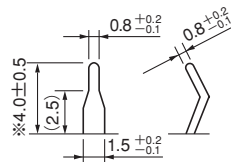
(端子形状)
