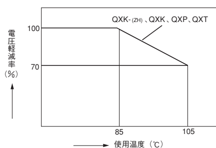
図1 電圧軽減と使用温度
