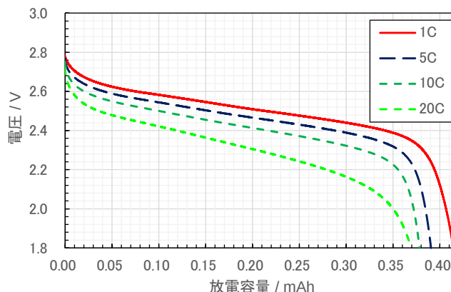
放電特性
