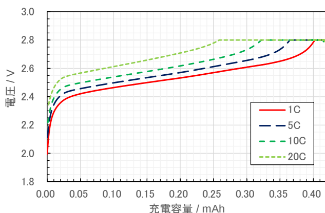
充電特性
