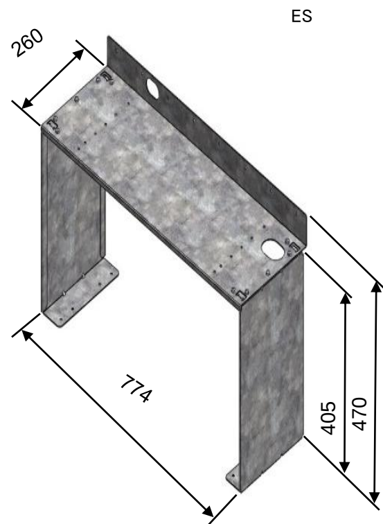
ラック単体のサイズ
