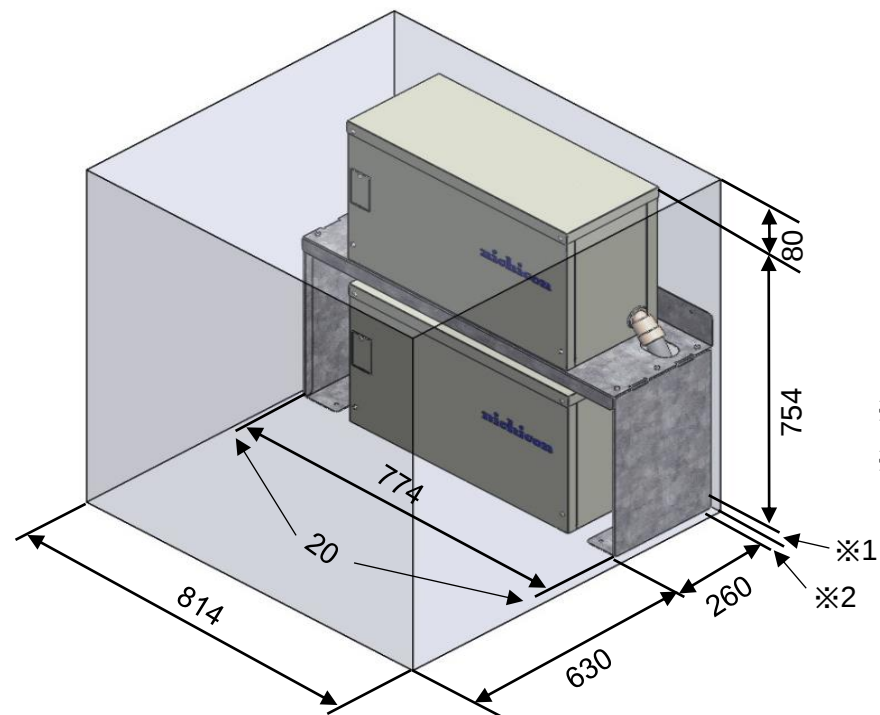
電池をセットした時のサイズと設置可能最少スペース
