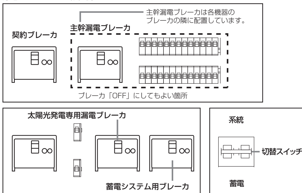
分電盤、ブレーカの配置例
