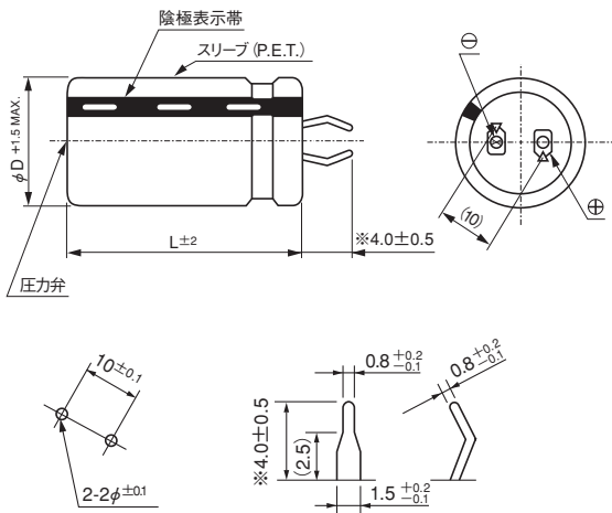
(基板穴寸法)
