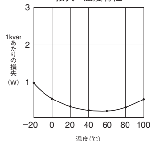
損失—温度特性
