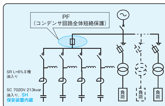
SH（蒸着電極）コンデンサご使用の場合（例） （[SH]・「保安装置内蔵」または「保護接点付き」）
