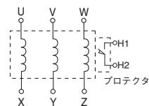
結線図
