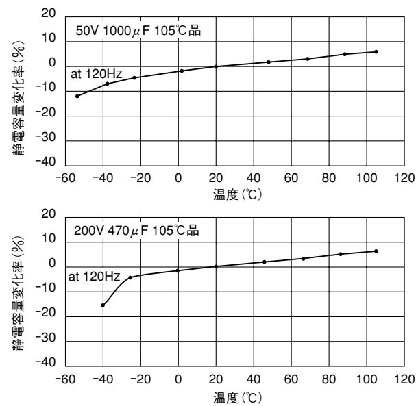
図 1-9 静電容量の温度特性
