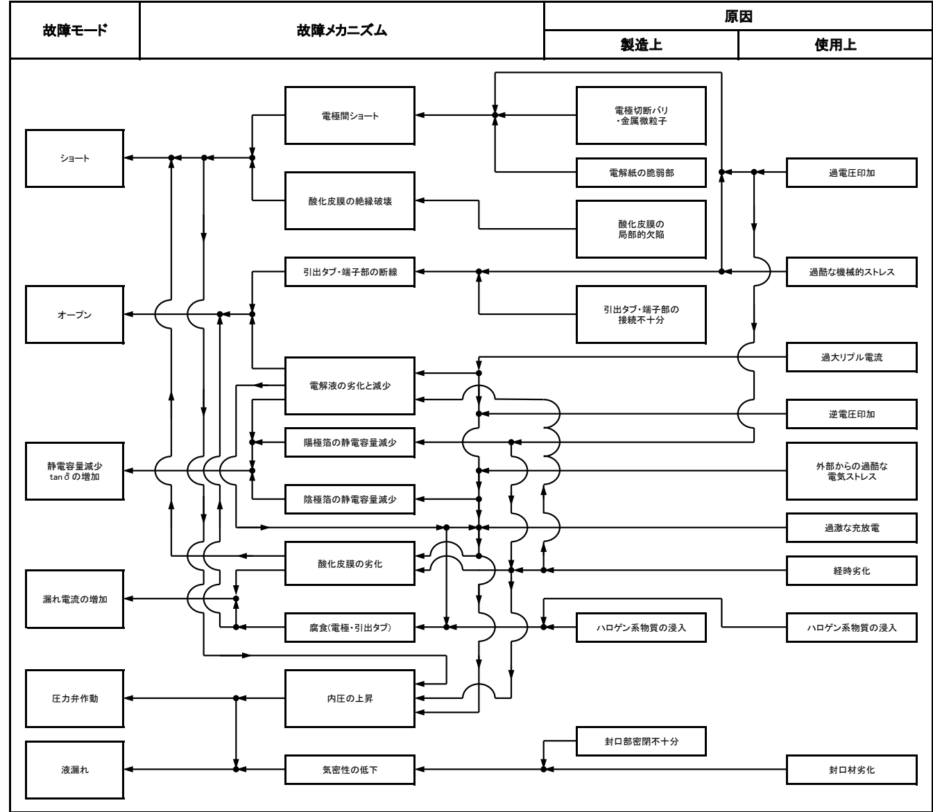
図 2-1 故障メカニズムの原因分析図
