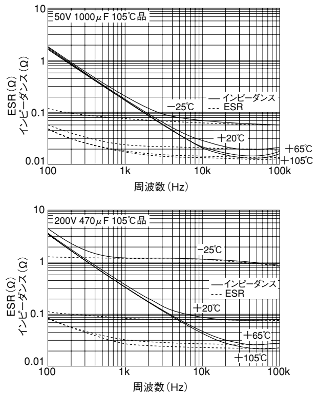
図 1-11 インピーダンス、ESRの周波数特性
