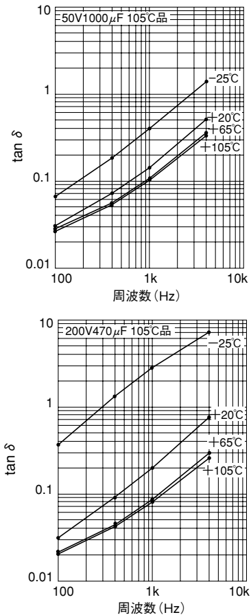
図 1-10 \tan \delta の周波数特性
