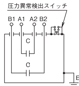
内部結線図
